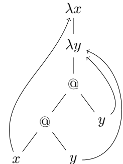
FIGURE 1 – arbre du terme \lambda xy.((x y) y)
